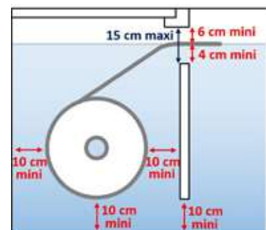
Cotas mínimas a respetar Cubiertas Sumergidas
