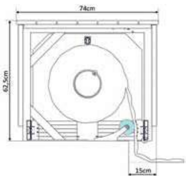
Dimensiones exteriores
