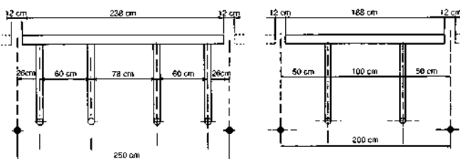
DETALLES DE ANCLAJE CUANDO LA MEDIDA «L» ES MAYOR 500 mm.
