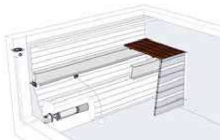
Playa sumergida motor en el eje (con anclajes)
