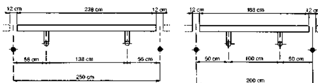
DETALLES DE ANCLAJE CUANDO LA MEDIDA «L» ES MENOR DE 500 mm.
