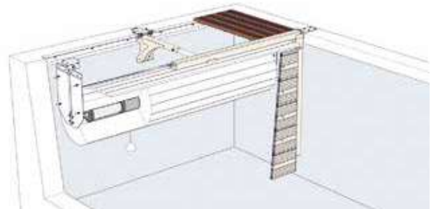
Motor en el eje fijación en pared
