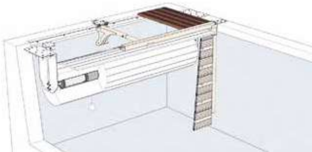
Motor en el eje fijación bajo piedra de coronación
