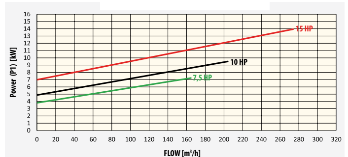
Potencia / Caudal
