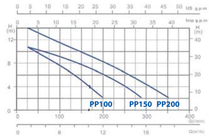
Curvas de rendimiento hidr ulico Hydraulic performance curves Courbes de performances hydrauliques Curve delle prestazioni idrauliche
