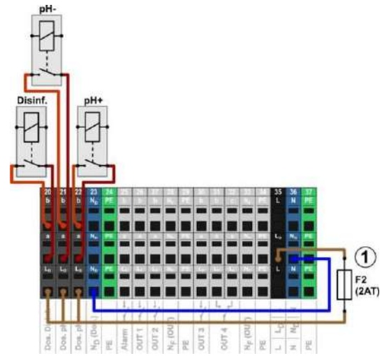
1 Fusible 2 AT para la fase LD a 230 V~ que alimenta las salidas de dosificación
