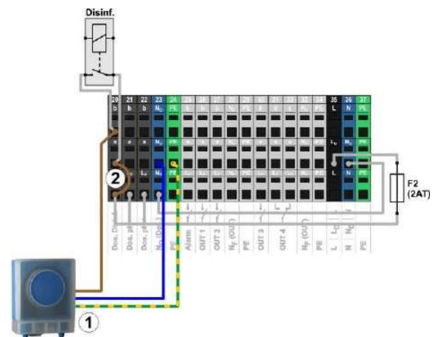
1 Bomba dosificadora estándar a 230 V~ (bomba peristáltica) 2 Puente en el compartimento de terminales de la fase LD al contacto central del relé 'a'
